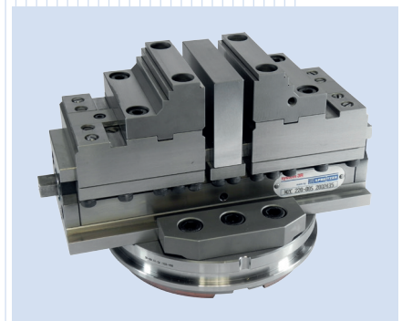
MZC 220-80 S mit Mittenbacke auf Palette MZC 220-80 S with center jaw on pallet
