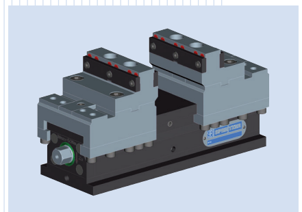
Mechanischer Zentrischspanner MZC mit Gripeinsätzen
