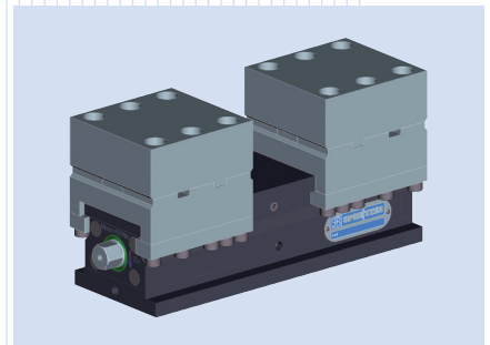
Mechanischer Zentrischspanner MZC mit weichen Blockbacken
