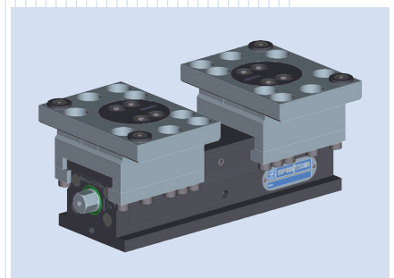
Mechanischer Zentrischspanner MZC mit Pendelbacken mit Gripeinsätzen
